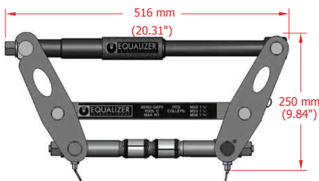
DIMENSIONES - ABIERTO
